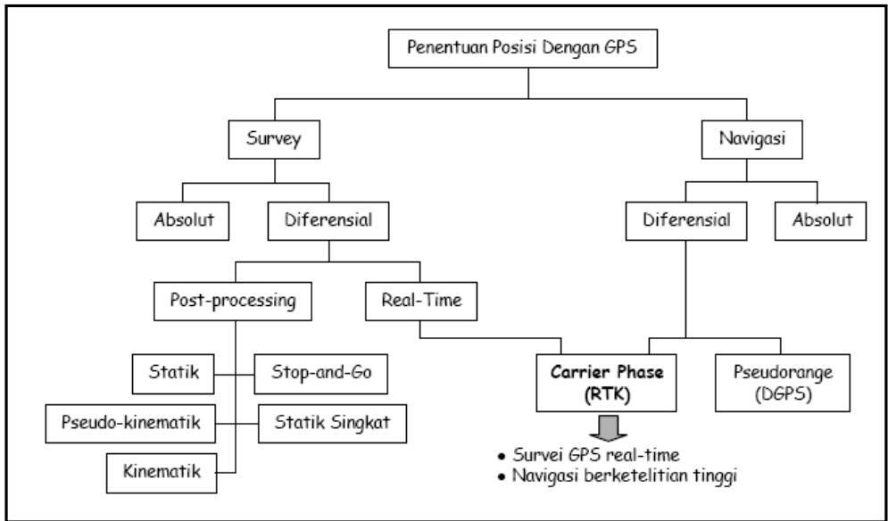
Gambar 2. Metode dan sistem penentuan posisi dengan GPS [Langley, 1998].
